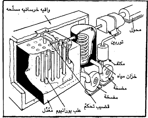
رسم توضيحي لجسم لمفاعل ذري - الفيزياء
